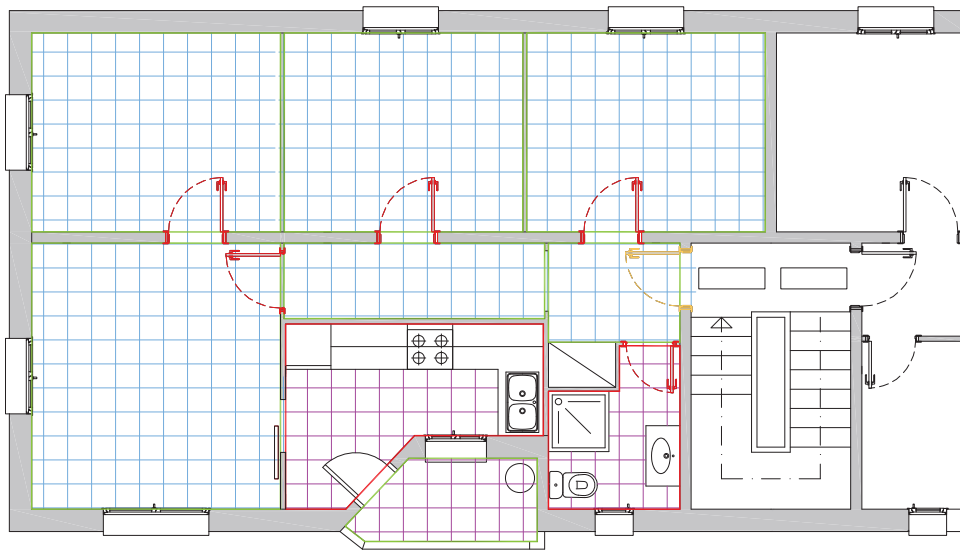
DETALL PAVIMENT
